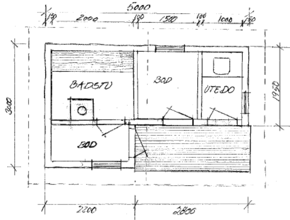
SITUASJONSPLAN H=1:50
